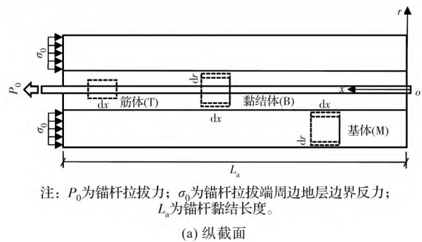
(a) 纵截面
