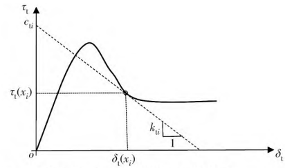
注: \tau_t 为界面剪应力; \delta_t 为界面剪切位移; k_t 为切线斜率; c_t 为切线的界面剪应力截距。
