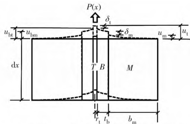
注: u_1 为筋体位移; u_{1b} 为黏结体在 T-B 界面的轴向位移; u_{1m} 为黏结体在 T-B 界面的轴向位移; u_m 为地层基体在 B-M 界面的轴向位移; \delta_t 为 T-B 界面的剪切位移; \delta_m 为 B-M 界面的剪切位移。
