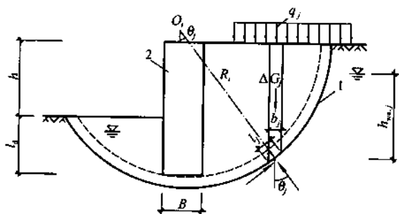
图 6.1.3 整体滑动稳定性验算
