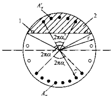
图 B.0.2 沿受拉区和受压区周边局部均匀配置纵向钢筋的圆形截面 1—构造钢筋; 2—混凝土受压区
