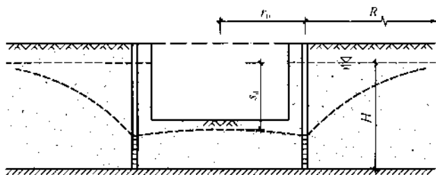
图 E.0.1 均质含水层潜水完整井的基坑涌水量计算
