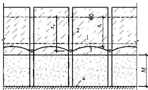
图 7.3.8 承压水完整井地下水水位降深计算
