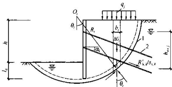
图 4.2.3 圆弧滑动条分法整体稳定性验算
