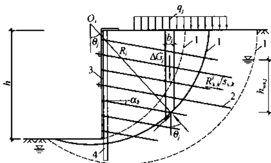
(b)水泥土桩或微型桩复合土钉墙
