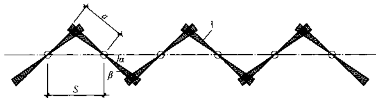
图6 摆喷帷幕平面形式
