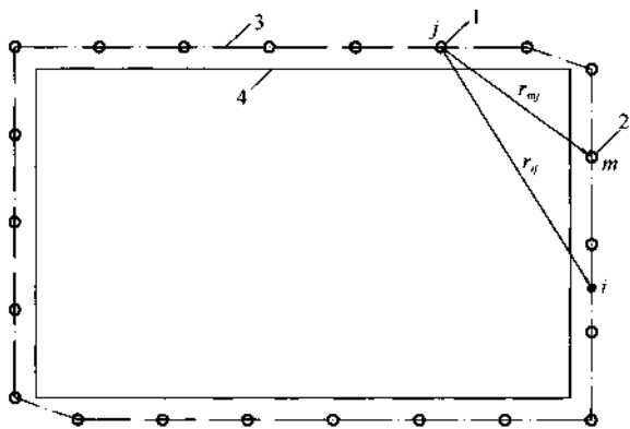
图 7.3.5-2 计算点与降水井的关系 1—第 j 口井; 2—第 m 口井; 3—降水井所围面积的边线; 4—基坑边线
