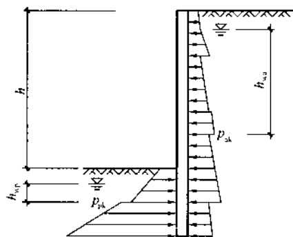
图 3.4.2 土压力计算
