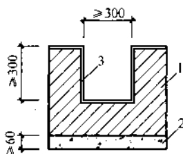
图8 排水明沟的截面及构造
