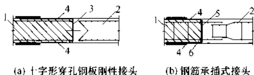
图2 地下连续墙刚性接头
