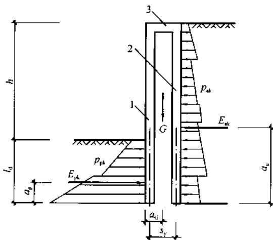
图 4.12.5 双排桩抗倾覆稳定性验算
