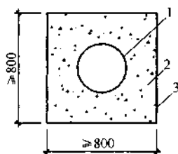
图9 排水盲沟的截面及构造
