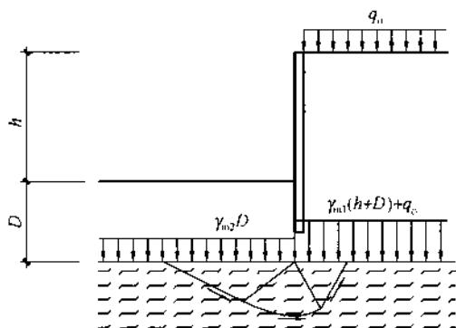
图 4.2.4-2 软弱下卧层的隆起稳定性验算
