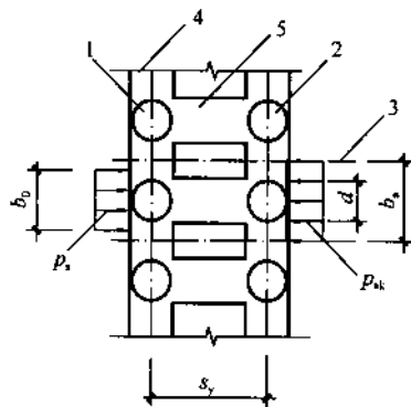
图 4.12.2 双排桩桩顶连梁及计算宽度
