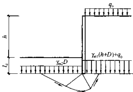
图 4.2.4-1 挡土构件底端平面下土的隆起稳定性验算
