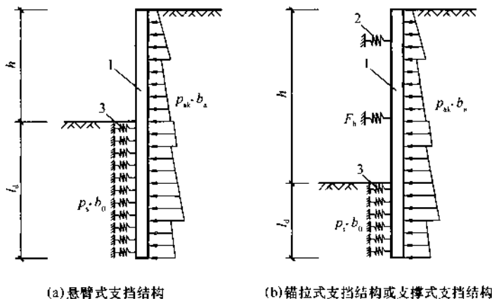
图 4.1.3-1 弹性支点法计算
