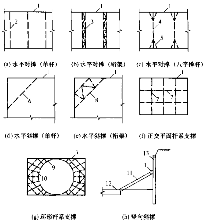
图4 内支撑结构常用类型
