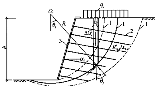
(a)土钉墙在地下水位以上
