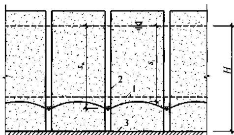
图 7.3.5-1 潜水完整井地下水位降深计算
