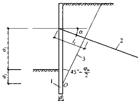
图 4.7.5 理论直线滑动面
