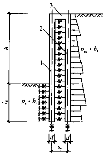
图 4.12.1 双排桩计算
