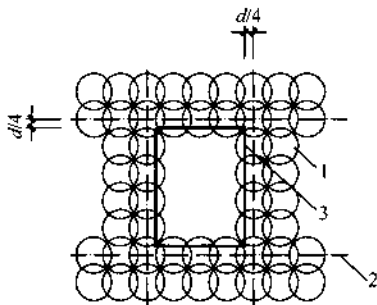
图 6.2.3 格栅式水泥土墙
