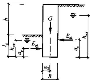
图 6.1.2 倾覆稳定性验算
