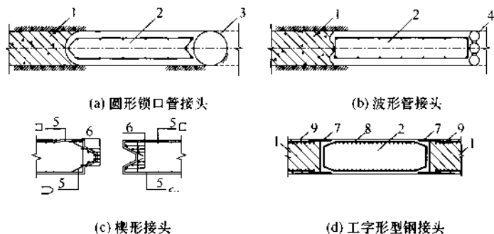
图1 地下连续墙柔性接头
