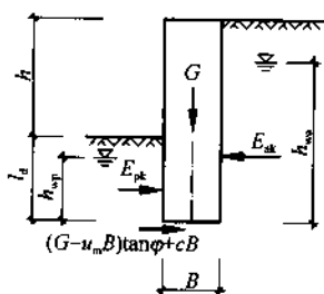
图 6.1.1 滑移稳定性验算
