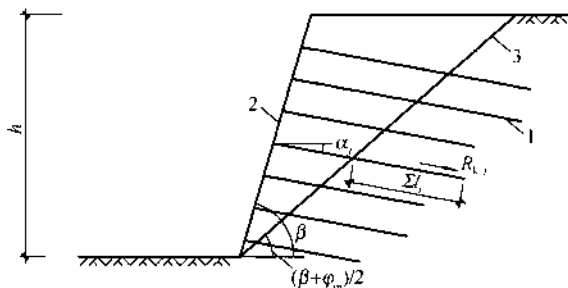
图 5.2.5 土钉抗拔承载力计算
