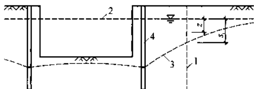
图 7.5.2 降水引起的附加有效应力计算
