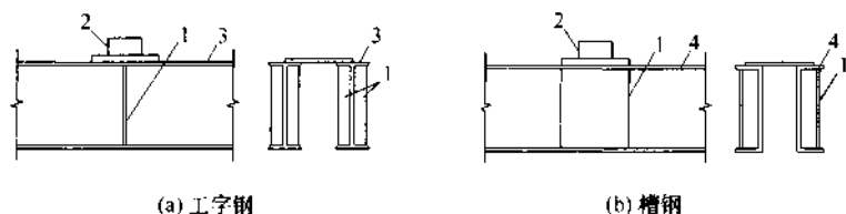
图3 钢腰梁的局部加强构造形式
