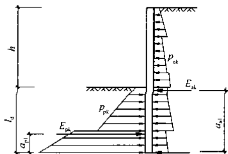
图 4.2.1 悬臂式结构嵌固稳定性验算
