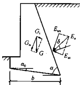
图 11.2.3 挡墙抗滑移稳定性验算
