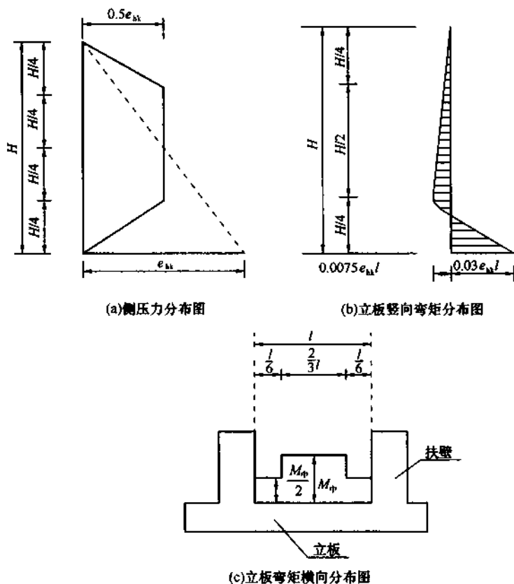
图 12.2.4 扶壁式挡墙侧向压力分布图
