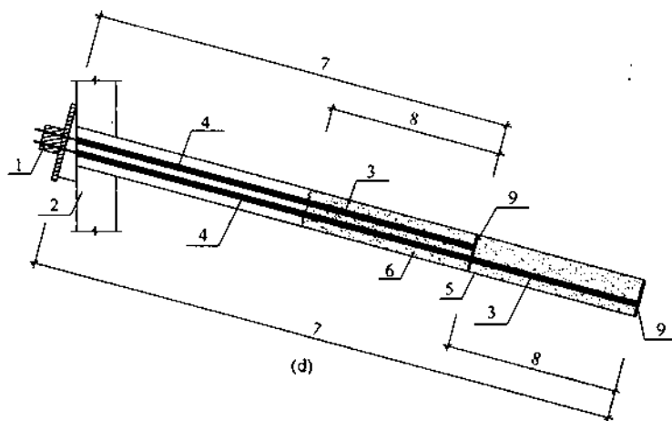
图2 压力分散型锚杆简图(二)
