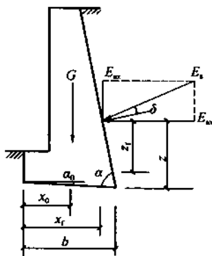
图 11.2.4 挡墙抗倾覆稳定性验算
