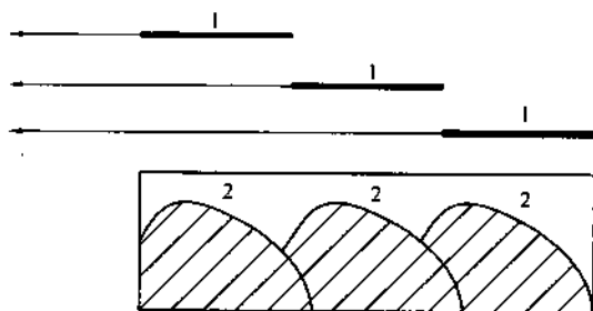
图5 荷载分散型锚杆锚固应力分布图
