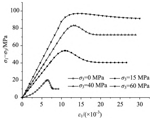
图 4 所提出模型理论曲线 (红砂岩)
