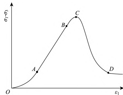
图 1 三轴压缩条件下空隙岩石变形破坏全过程
