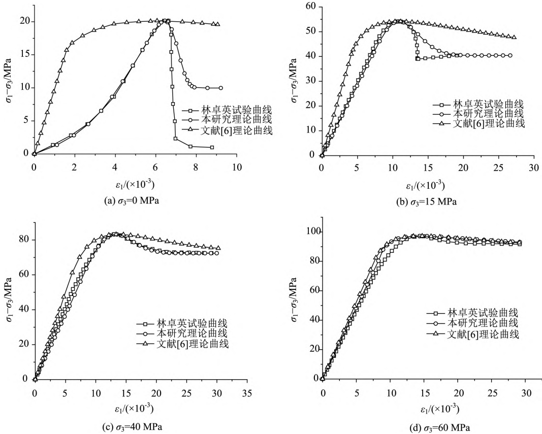
图 5 红砂岩试验曲线与理论曲线比较
