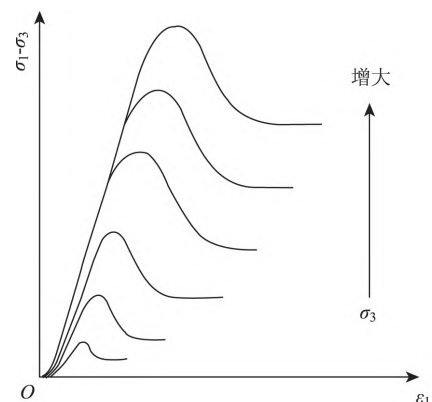
图 2 不同围压作用下空隙岩石变形破坏全过程
