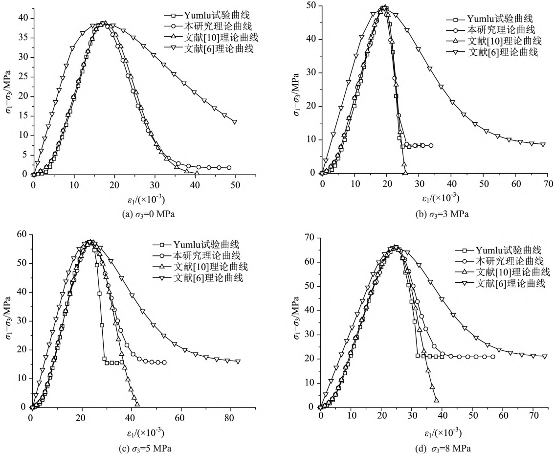
图 6 煤岩试验曲线与理论曲线比较
