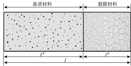
图3 空隙岩石非线性变形细观唯象分析模型
